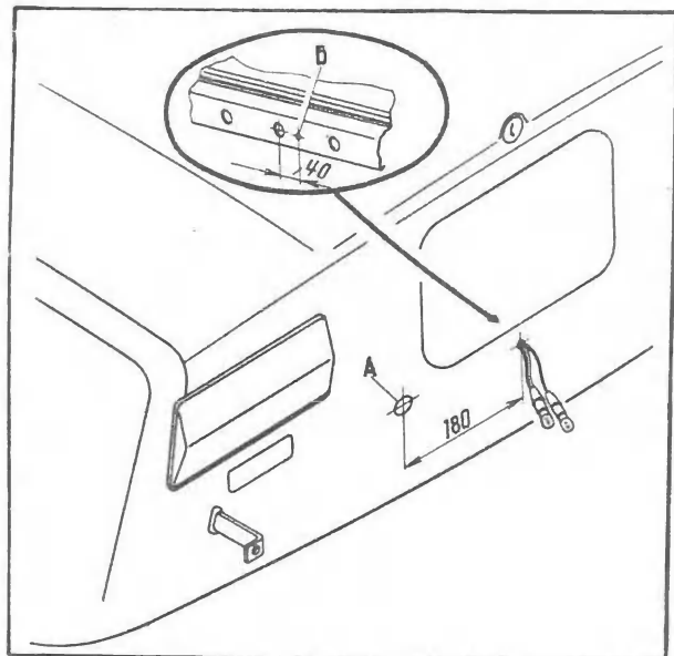
Рис. 3. Схема подключения дополнительного пучка проводов к электропроводке автомобиля (провода автомобиля показаны тонкими линиями): 48 — плафон освещения кузова; 50 — лампа освещения багажника; 51 — задние фонари; 52 — фонарь номерного знака; 53 — штепсельная розетка; 54 — выключатель указателей поворота в задних фонарях автомобиля. Обозначения цвета проводов: Б — белый; Г — голубой; Ж — желтый; К — красный; Кор — коричневый; Ч — черный; ГЧ — голубой с черными полосками. Нумерация приборов та же, что в инструкции.
